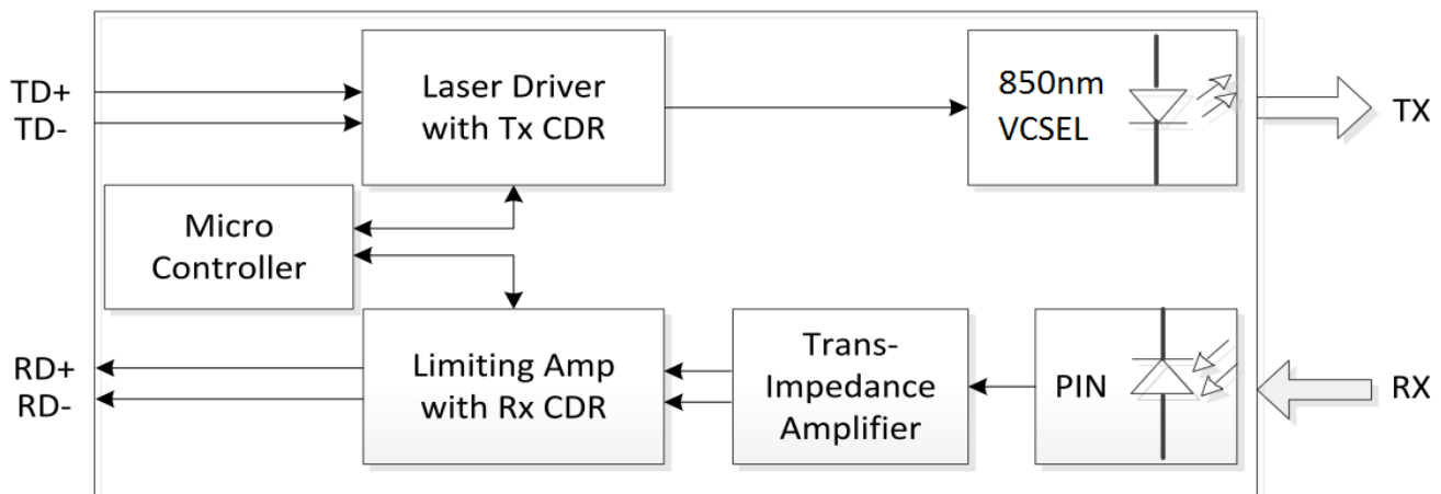
SFP28 SR Module
